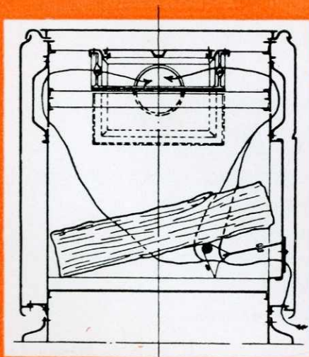
Vue en coupe montrant la distribution de l'air de combustion grâce au chenet spécial, et le circuit des flammes jusqu'à la buse de départ.
